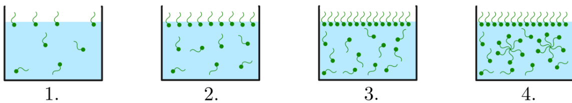
FIGURE 1.5: Schéma de solubilité d'un tensioactif. On a représenté quatre concentrations en tensioactifs pour le cas de tensioactifs insolubles (en rouge) et solubles (en vert). Les concentrations augmentent du schéma 1. au 4.. À forte concentration, on observe l'apparition d'une bi-couche de tensioactifs pour les tensioactifs insolubles, et l'apparition de micelles pour les tensioactifs solubles [49].
